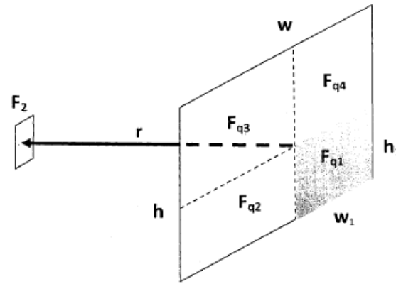
Рисунок А.3.1. Расположение излучающей поверхности пламени F_1 и облучаемой поверхности материала соседнего объекта F_2 , где w и h - соответственно длина и ширина поверхности пламени.
